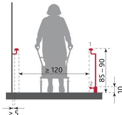
34 Rampe, Querschnitt
