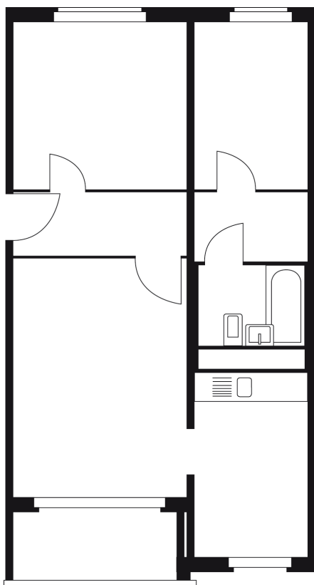
Grundriss Bestand
